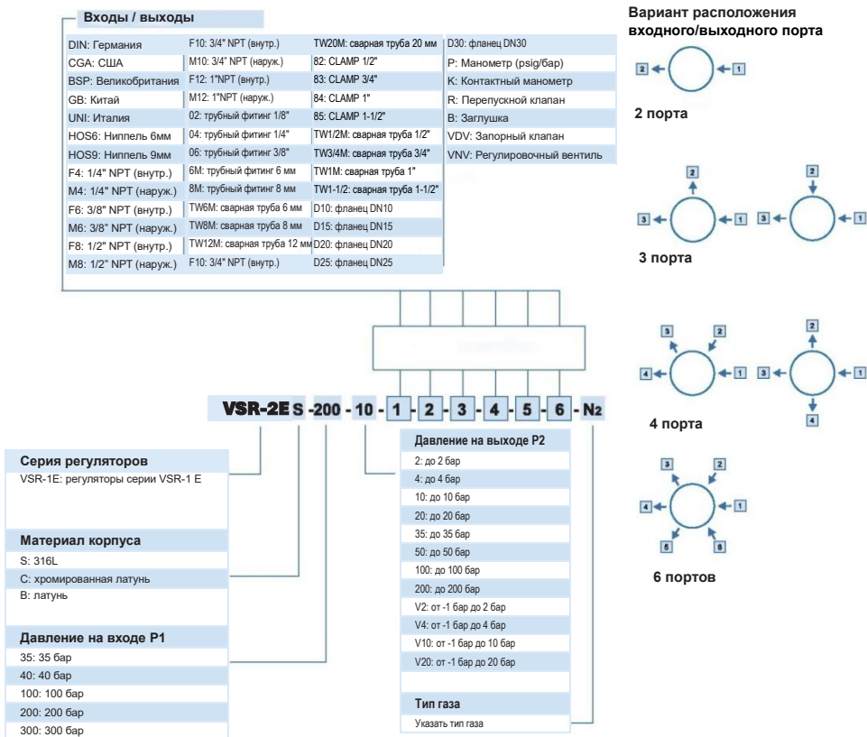
Рис. 3 Конфигуратор характеристик регулятора
