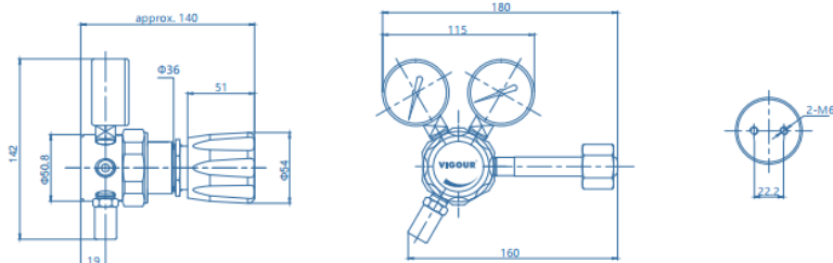
Рис.1 Габаритные размеры
