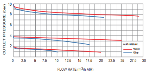
Рис.2 График потока
