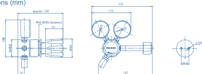
Рис.1 Габаритные размеры
