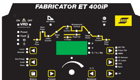
Панель управления Fabricator ET 400iP
