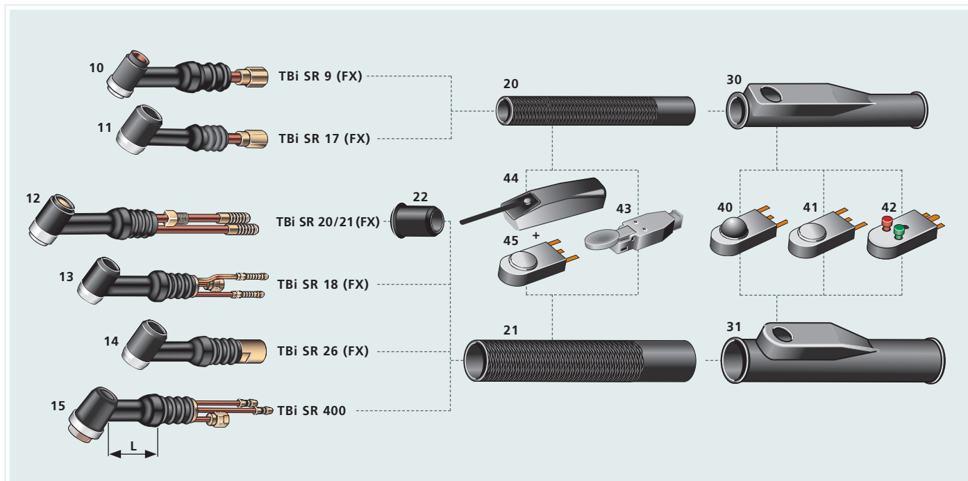
Рукоятки и кнопки / Handle tubes and switches / Poignées tubulaires et gâchettes
