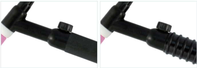
Рукоятки для горелок с вентилем / Handle tubes for torch bodies with valve / Poignées pour version à valve
