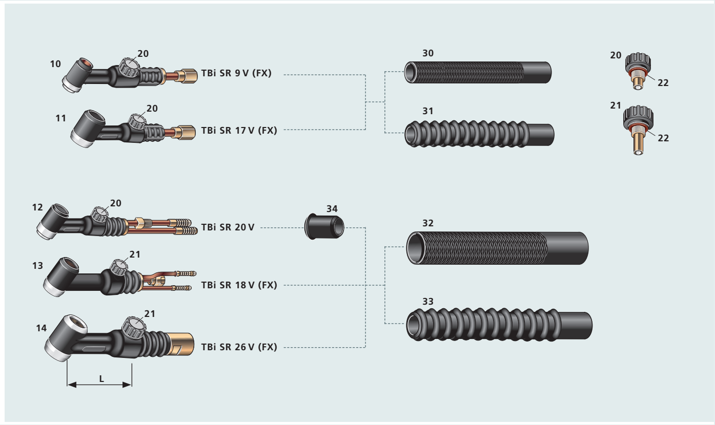
Рукоятки для горелок с вентилем / Handle tubes for torch bodies with valve / Poignées pour version à valve
